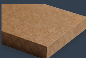
333 - Adobe
