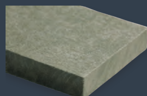
050 - Grafite
