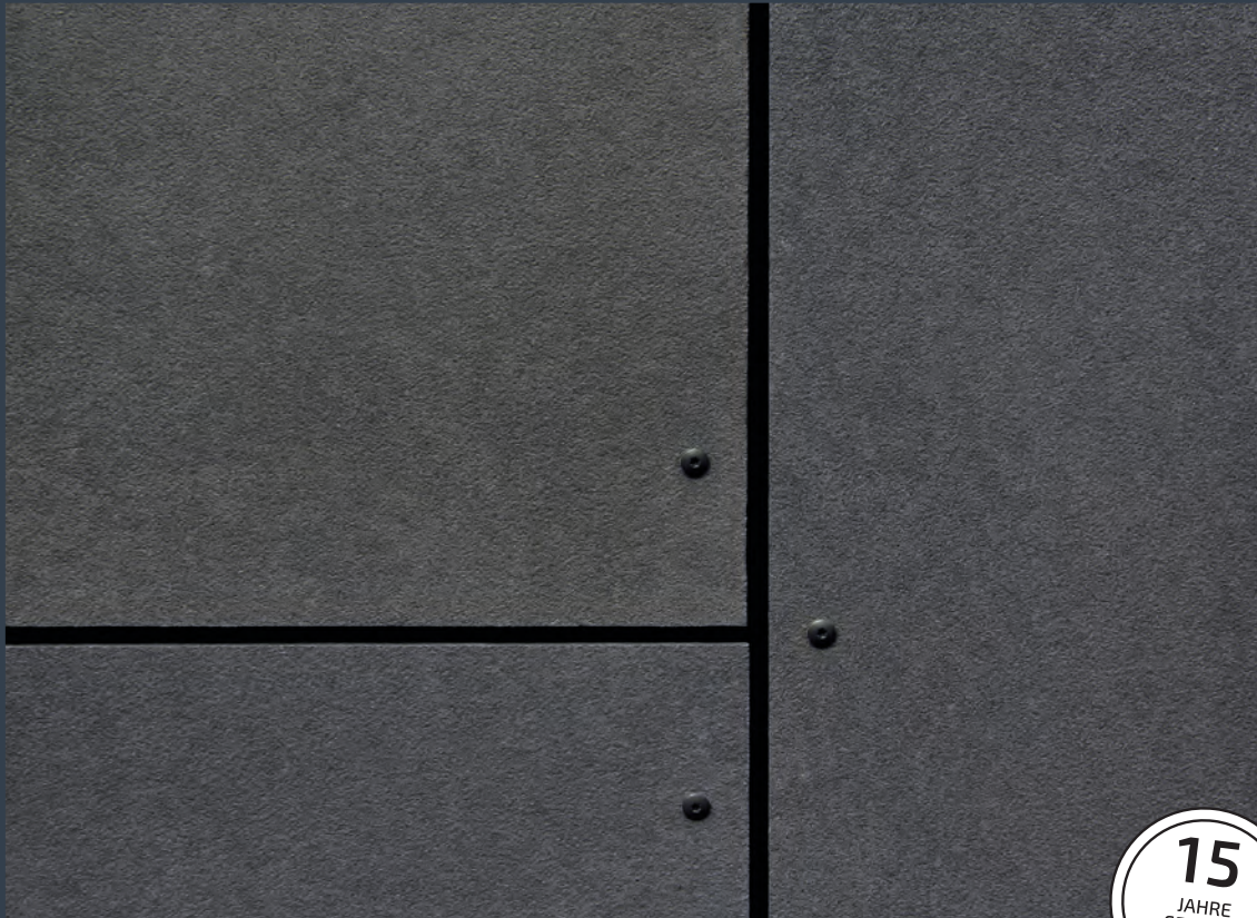
070r - Flint
