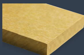
565 - Amber
