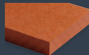
343 - Ruby
