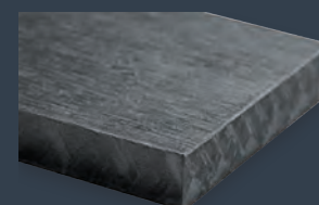
070 - Flint
