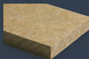
313 - Tufa
