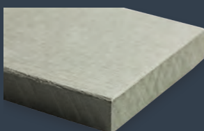
020 - Granite
